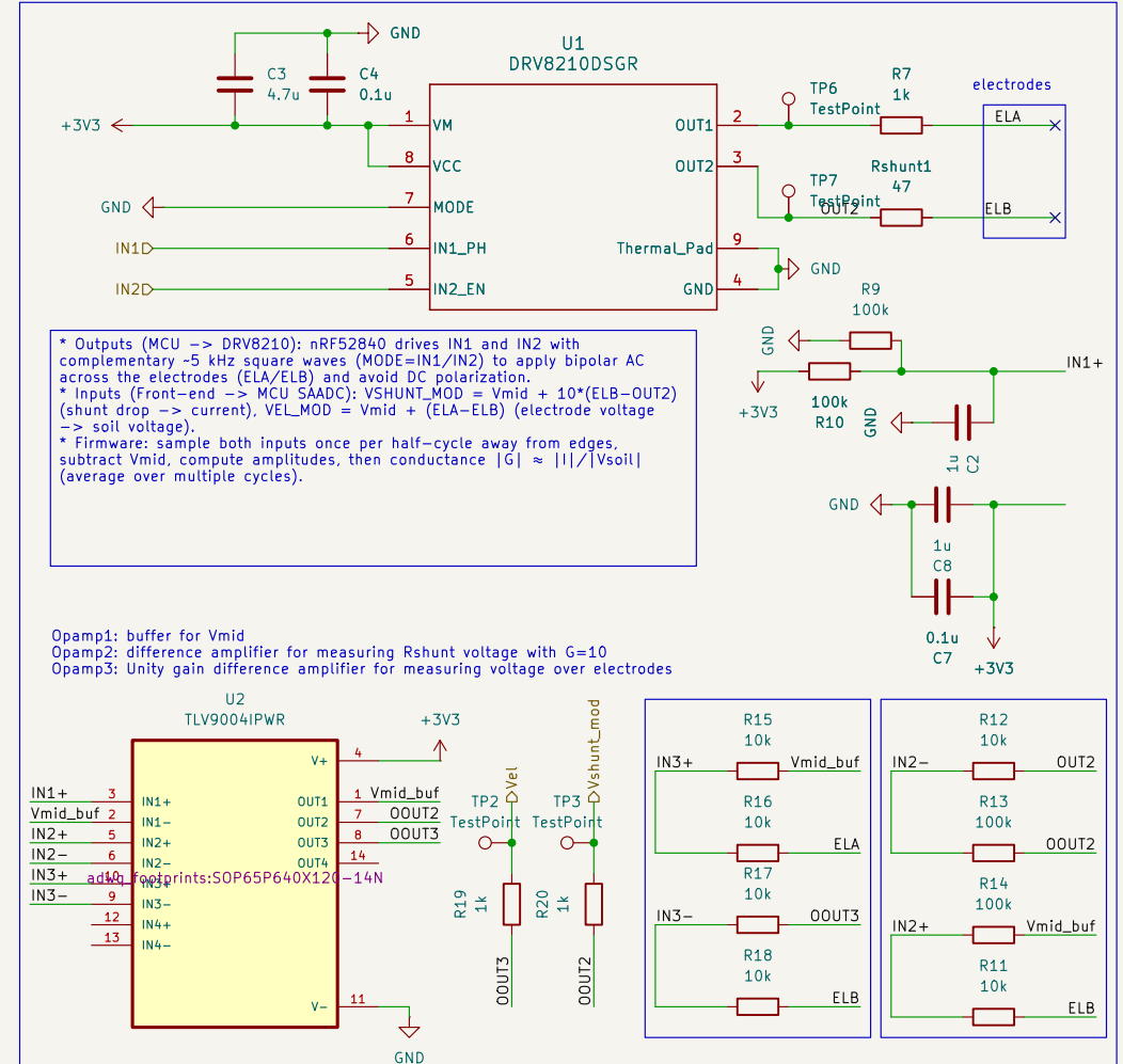
EC sensor 5KHz
